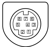
Klemmenanordnung
